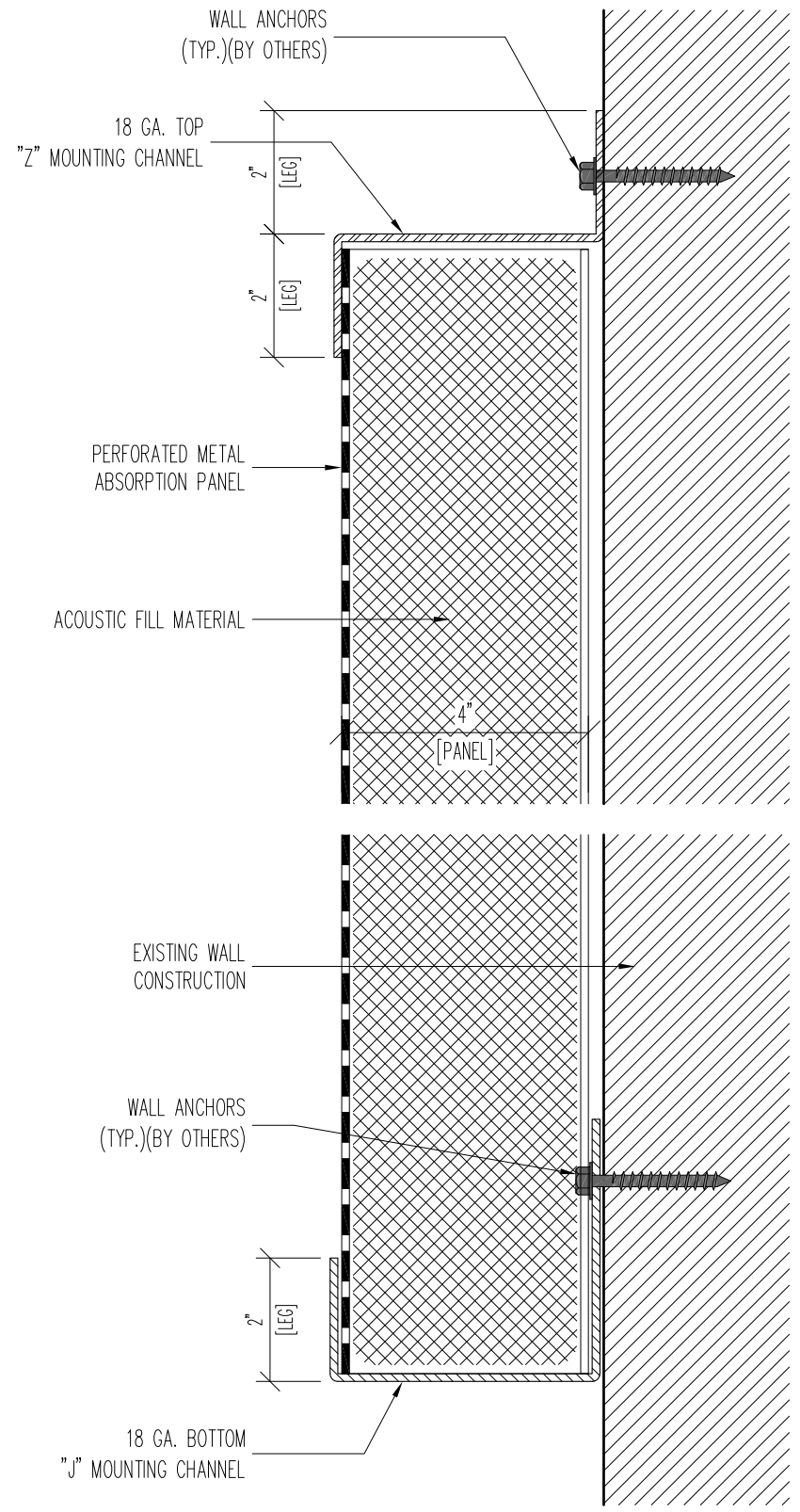
SECTION A-A
