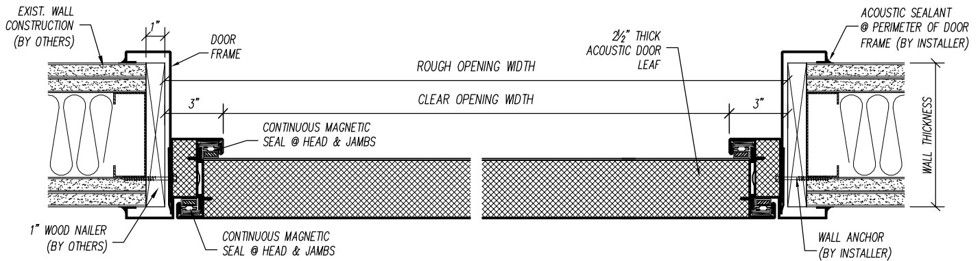
JAMB DETAIL
